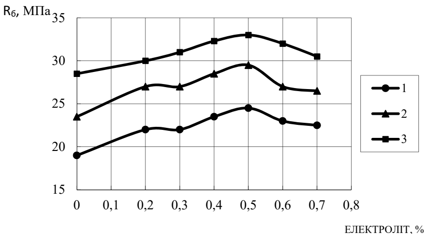
Рис. 1. межа міцності золотшлакового вакуумбетону залежно від витрати електроліту: 1 – при витратах цементу 280 кг/м 3 ; 2 – теж, при 350 кг/м 3 ; 3 – теж, при 400 кг/м 3
