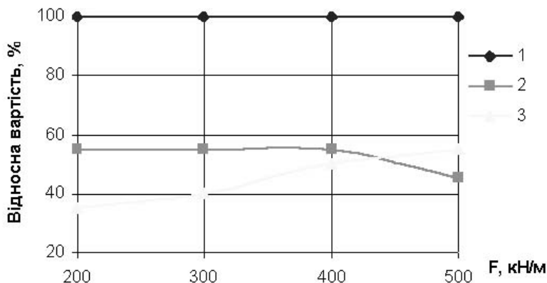
Рис.3. Графік відносної вартості стрічкових фундаментів залежно від діючого на них вертикального навантаження: 1 – для пальових фундаментів традиційної конструкції; 2 – для пальових фундаментів з подушкою під ростверком; 3 – для фундаментів неглибокого закладення
