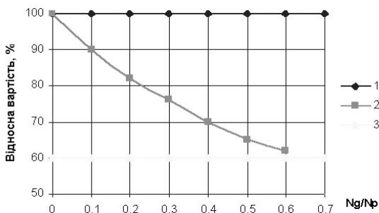
Рис.2. Графіки відносної вартості стрічкових фундаментів залежно від їх конструктивного вирішення: 1 – для пальових фундаментів традиційної конструкції; 2 – для пальових фундаментів з подушкою під ростверком; 3 – для фундаментів неглибокого закладення; N_g – частина вертикального навантаження, що передається на ґрунти основи через підшову ростверка; N_p – те ж, через палі
