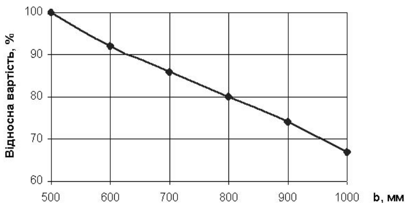
Рис.4. Графік залежності відносної вартості пальових фундаментів з подушкою під ростверком, що мають різну ширину підшви b
