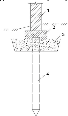
Рис.1. Поперечний переріз стрічкового пальового фундаменту з подушкою під ростверком: 1 – стіна будівлі; 2 – стрічковий залізобетонний ростверк фундаменту; 3 – подушка з сипучих матеріалів; 4 – залізобетонні палі
