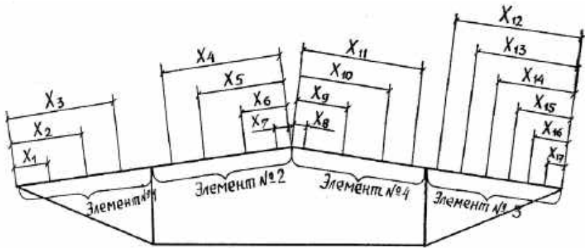
Рис. 9. X-координати перерізів верхнього пояса з встановленими тензорезисторами
