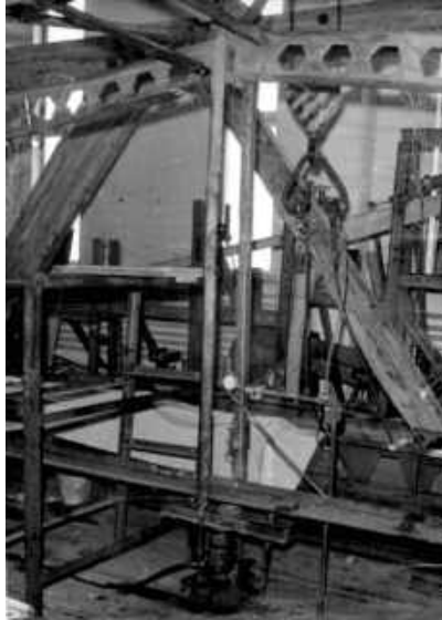
Рис. 5. Система передачі навантаження на коньковий вузол
