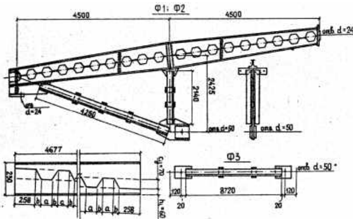
Рис. 3. Відправні марки ферми
