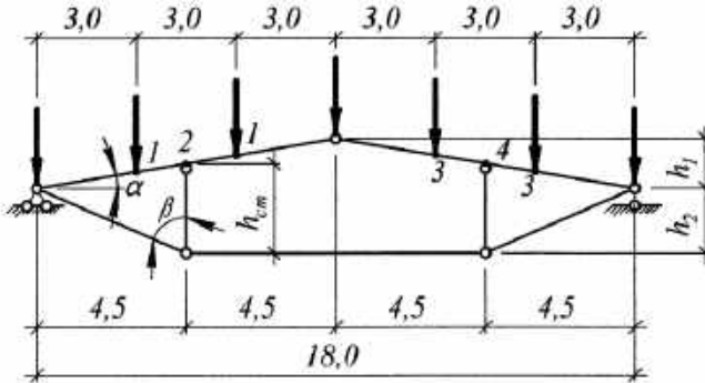
Рис.1. Вихідна система ферми
