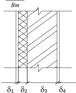
Рис.1. Конструкція стіни
